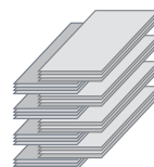
Auto-shift sorting/grouping
